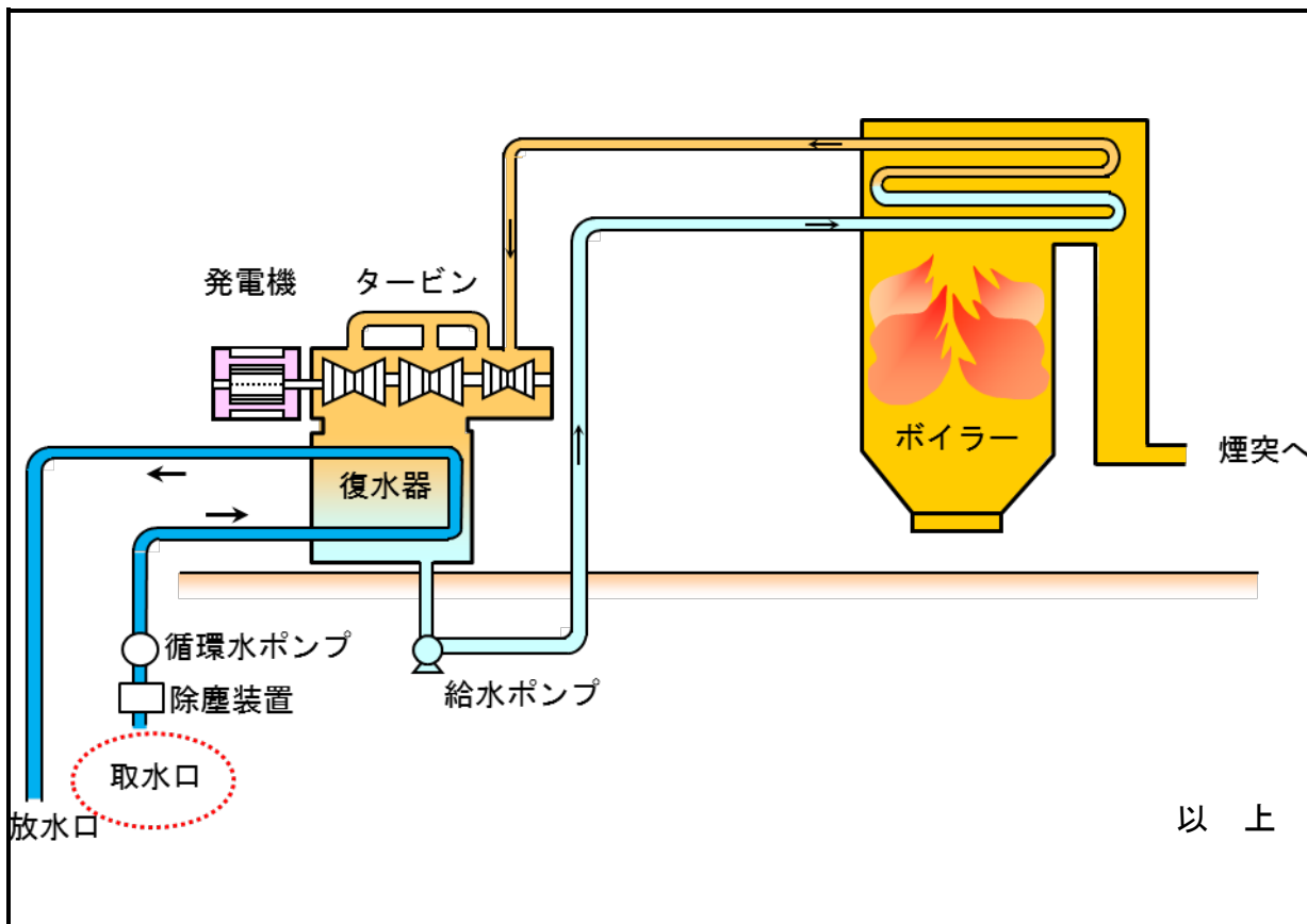
【富山新港火力発電所 1号機概要図】
