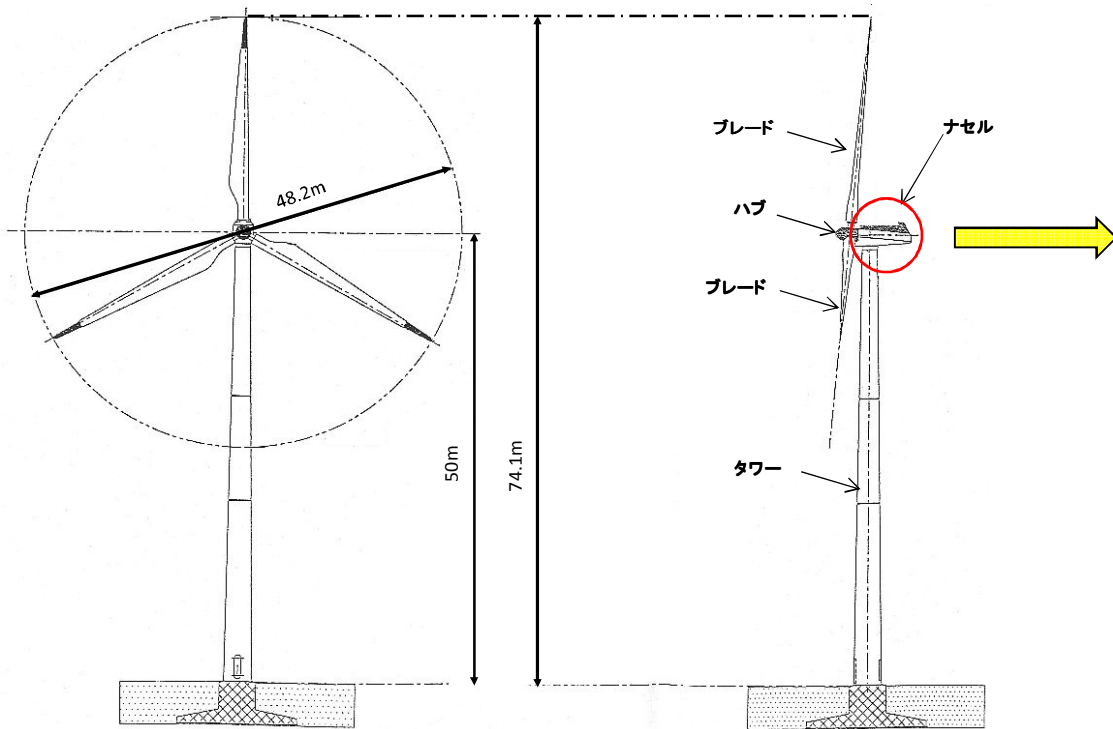
風車外形図
