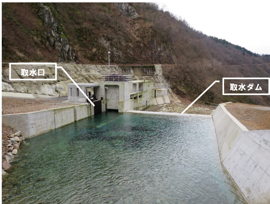
取水設備周辺 (取水ダム上流側より)
