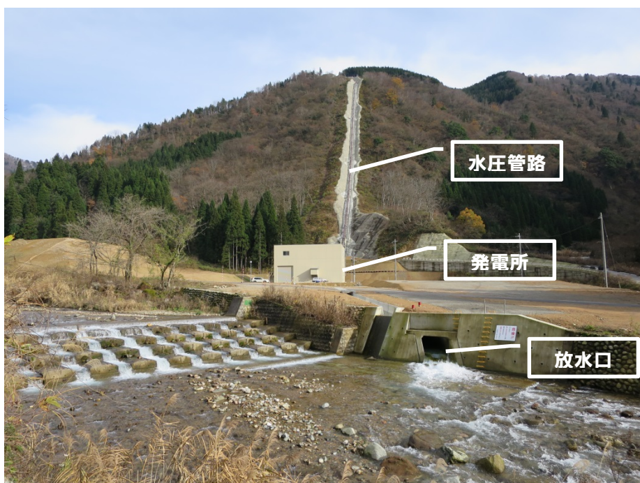
水圧管路～発電所周辺 (放水口対岸より)
