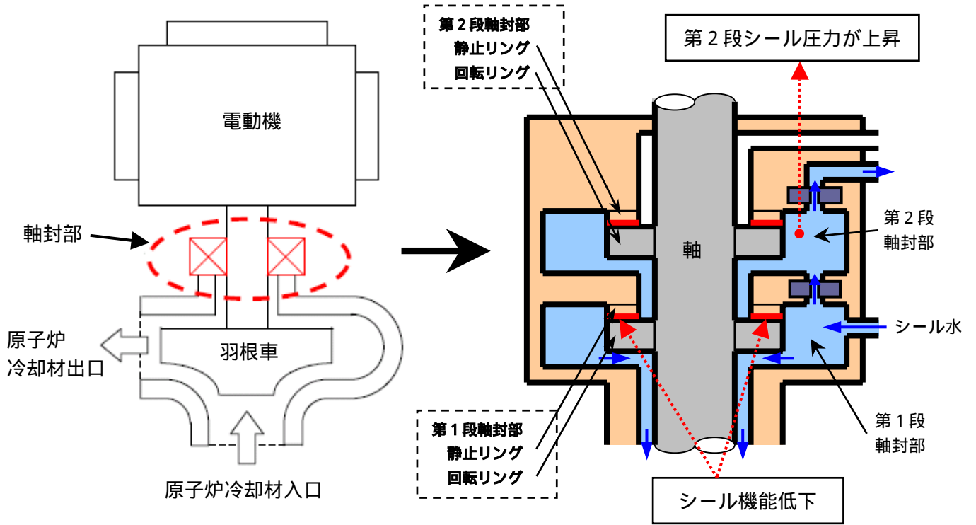
軸封部拡大図
