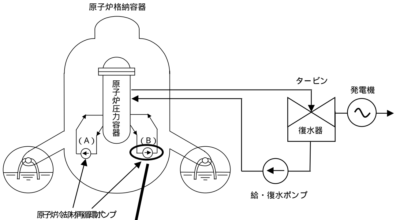
系統概要図
